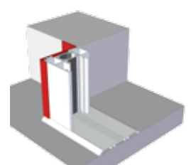
C: Montageprofil hinter der Fassade
